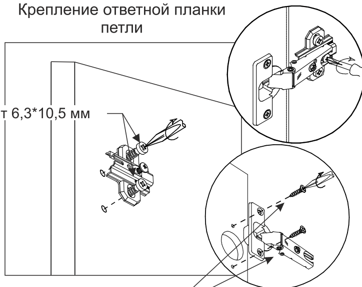
Шуруп универ 4*13 мм
