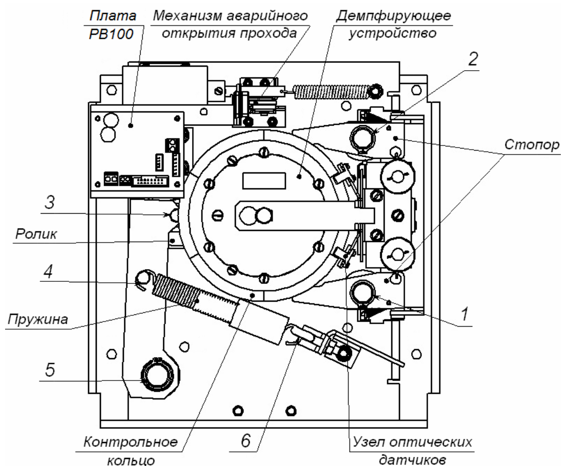
Рисунок 14. Расположение внутренних деталей и узлов стойки ЭП
