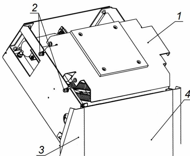
Рисунок 12. Стойка ЭП со снятой крышкой
