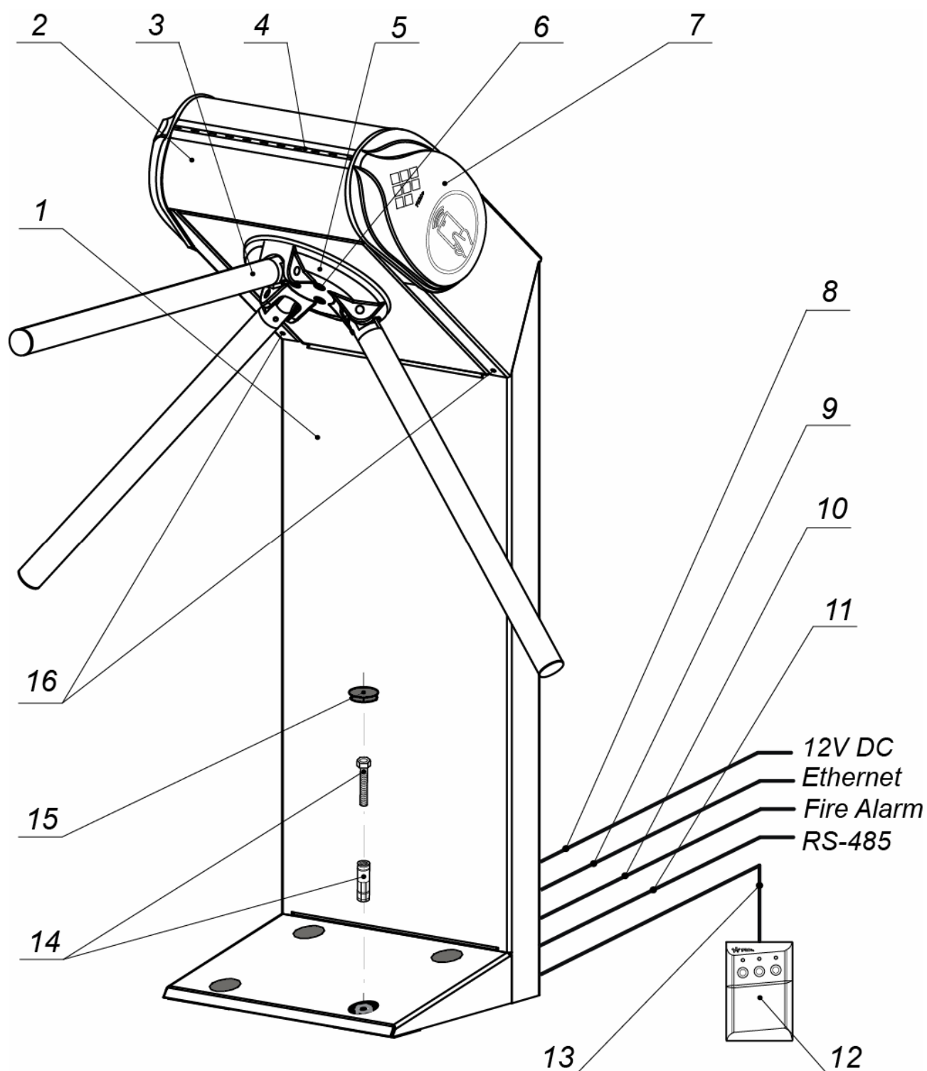
Рисунок 2. Устройство ЭП:
