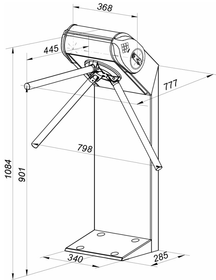
Рисунок 1. Габаритные размеры ЭП
