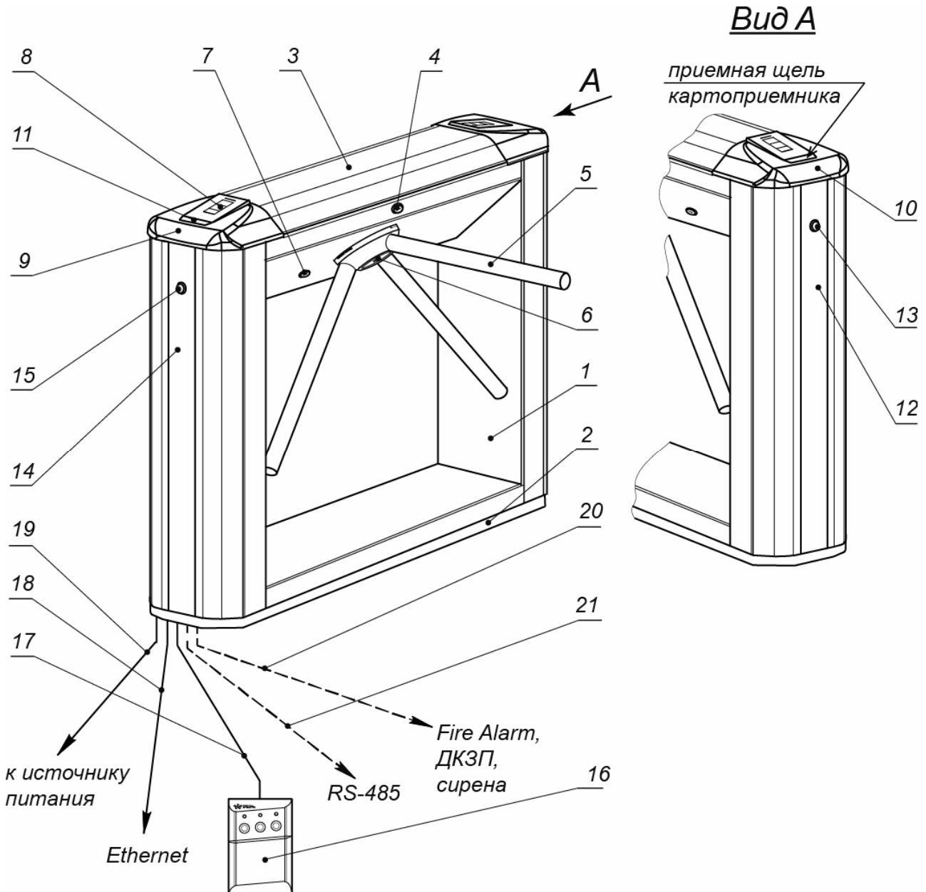
Рисунок 1. Устройство ЭП
