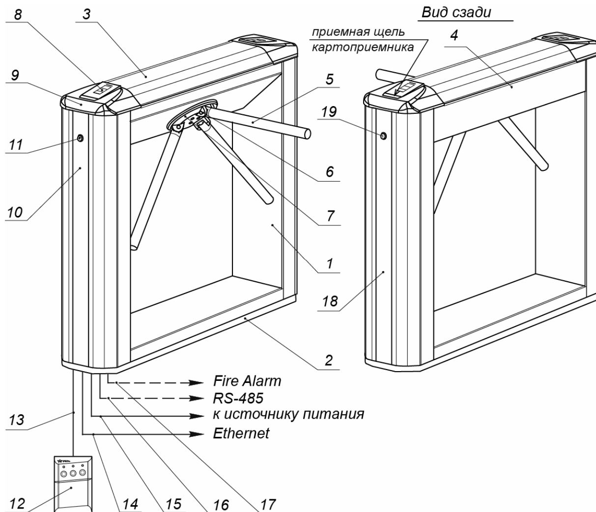
Рисунок 2. Устройство ЭП
