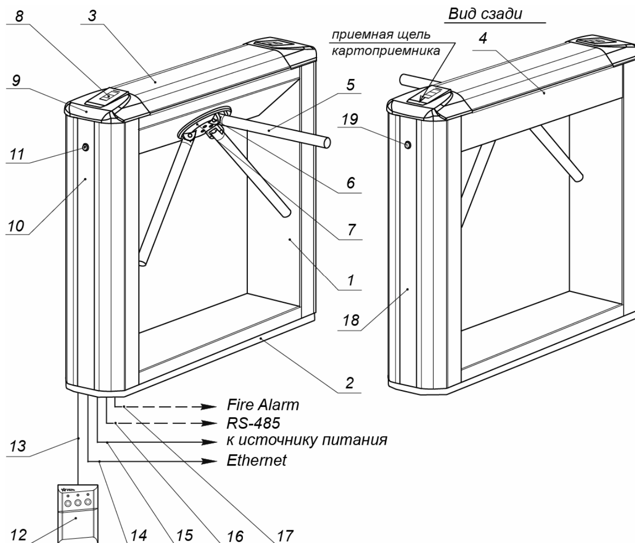
Рисунок 1. Устройство ЭП
