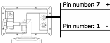
Power/Data cable
