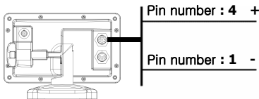
Power/Data cable
