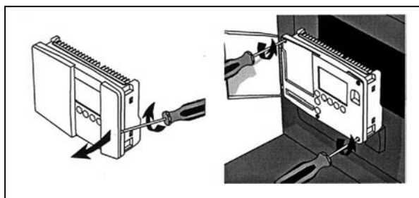
Рис. 24а. Установка корпуса в шкаф управления.
