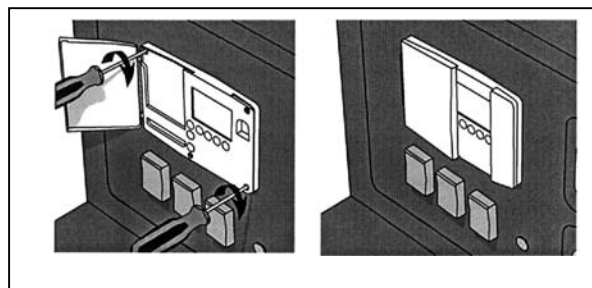
Рис. 24б. Установка корпуса в шкаф управления.
