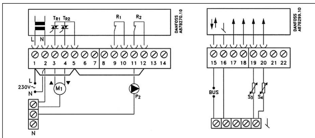
Рис. 13. Схема электрического соединения на 230 В к рис.3-5.
