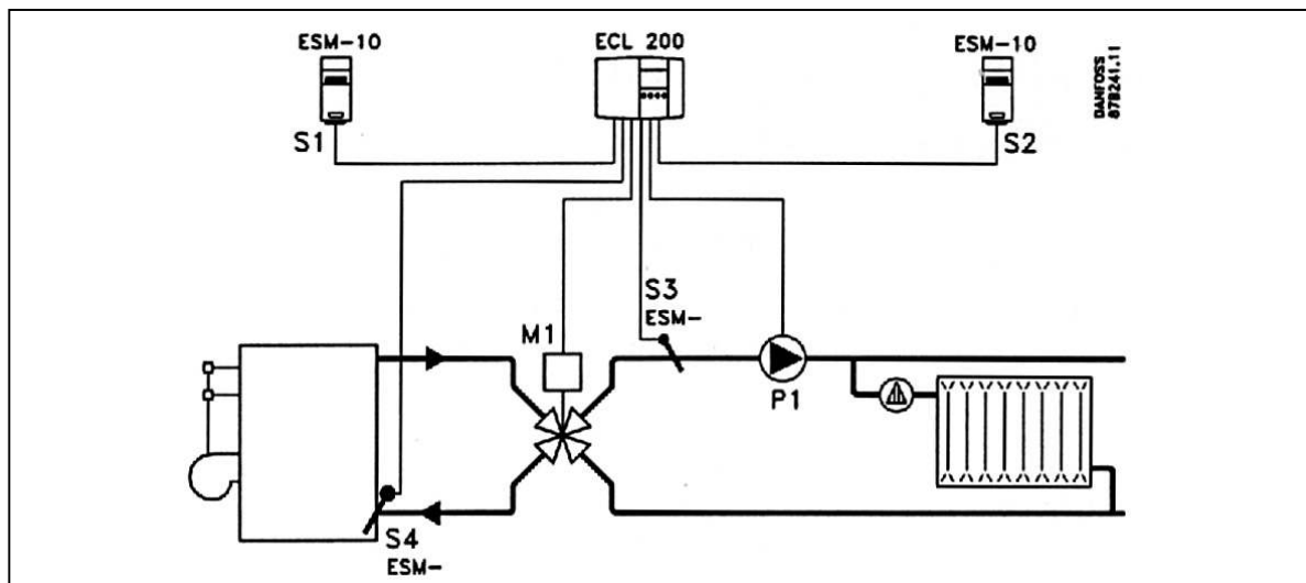
Рис. 12. Схема применения –4.
