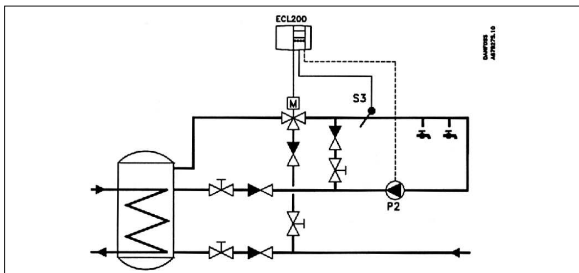
Рис. 5. Схема применения – 3.
