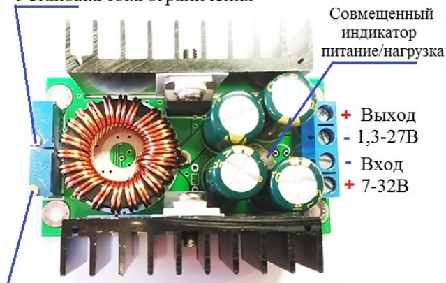
Эскиз подключения. Рис. 2
