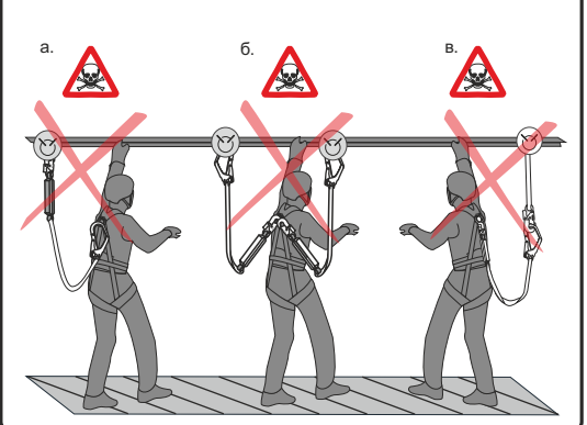
Рис. 10. Способы крепления стропов к анкерным устройствам
