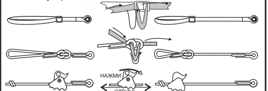
Рис. 11. Регулировка длины
