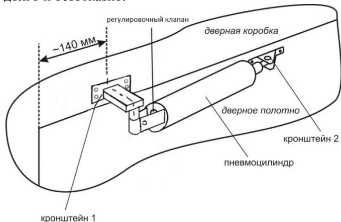
Рис. 1 – общий вид доводчика, когда дверь открывается наружу
