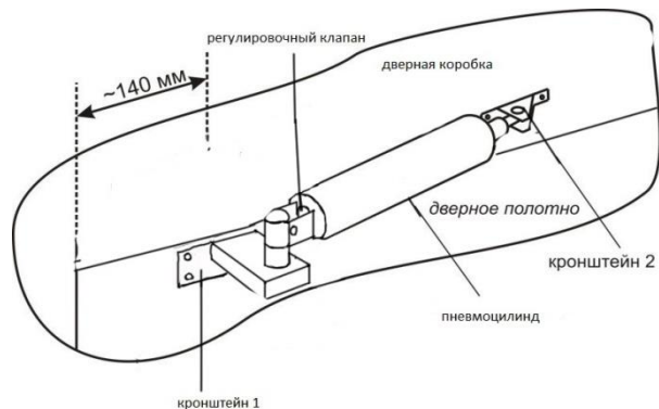
Рис. 1 – общий вид доводчика, когда дверь открывается наружу
