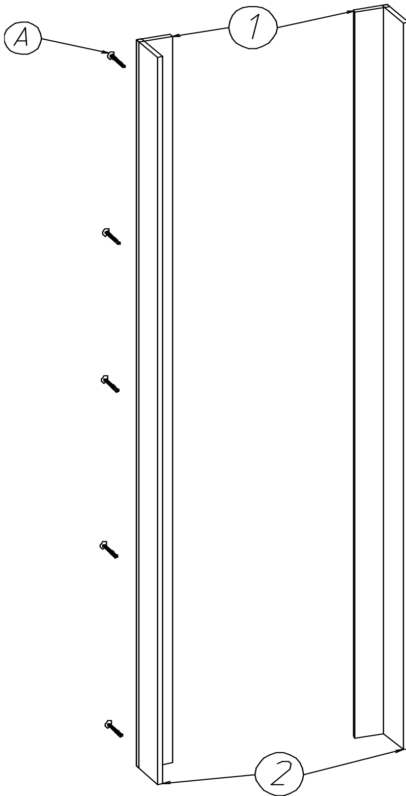
КС-101 Боковые стойки 2416x100x146
