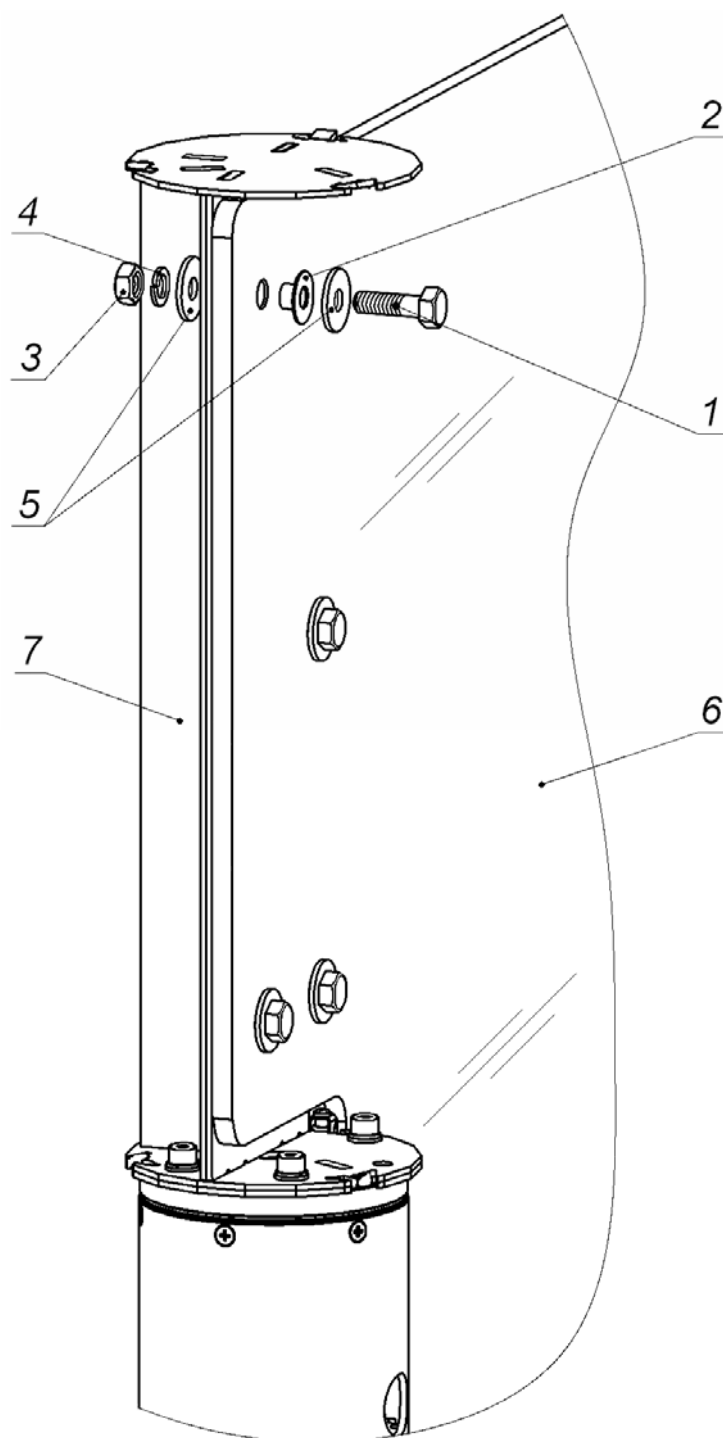
Рисунок 12. Установка створки
