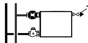
Рис. 1.7. Установка воздухоотводчика (1) на радиаторе
