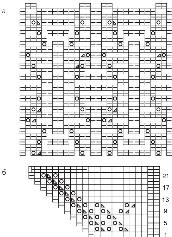
Рис. 6. Схемы узоров для вязания квадратной шали: а – для основного полотна (схема 1); б – для зубчатой каймы (схема 2)
