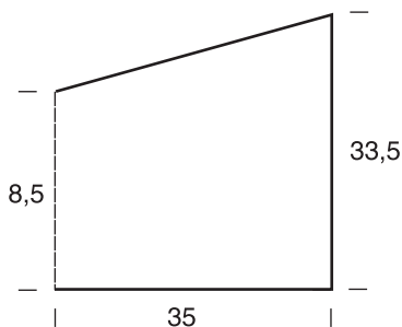
Рис. 21. Выкройка шали (1/2 изделия)
